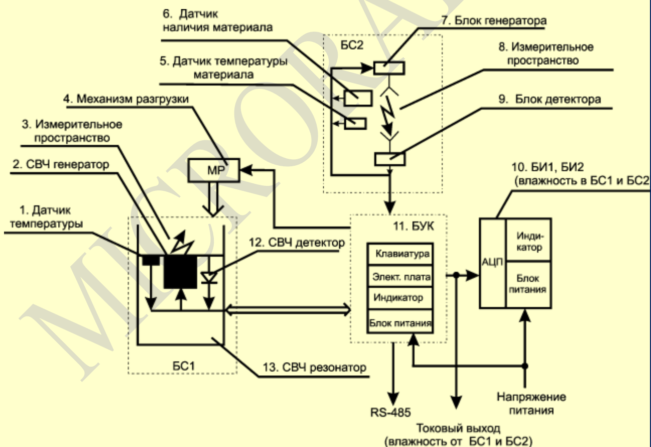
Рис. 6.1. Функциональная схема влагомера «Микрорадар-125»
