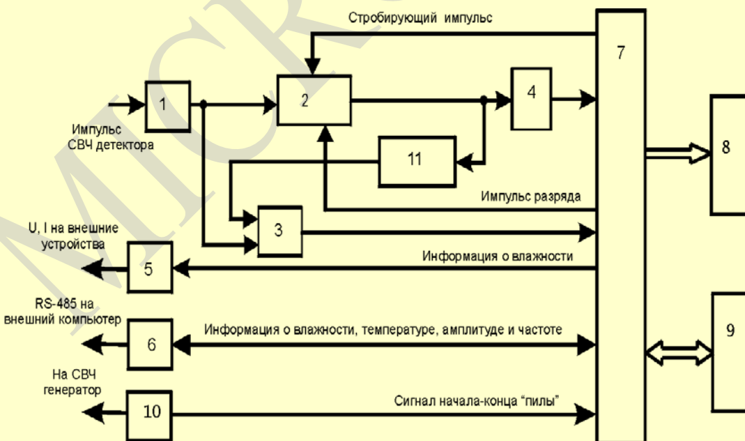
Рис. 4.1. Функциональная схема БУК влагомера «Микрорадар-114**»
