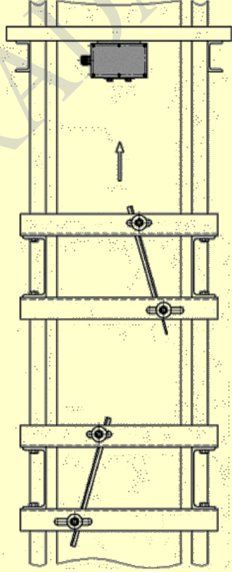
УСТАНОВКА ФОРМИРОВАТЕЛЕЙ ПОТОКА. ОБЩИЙ ВИД
