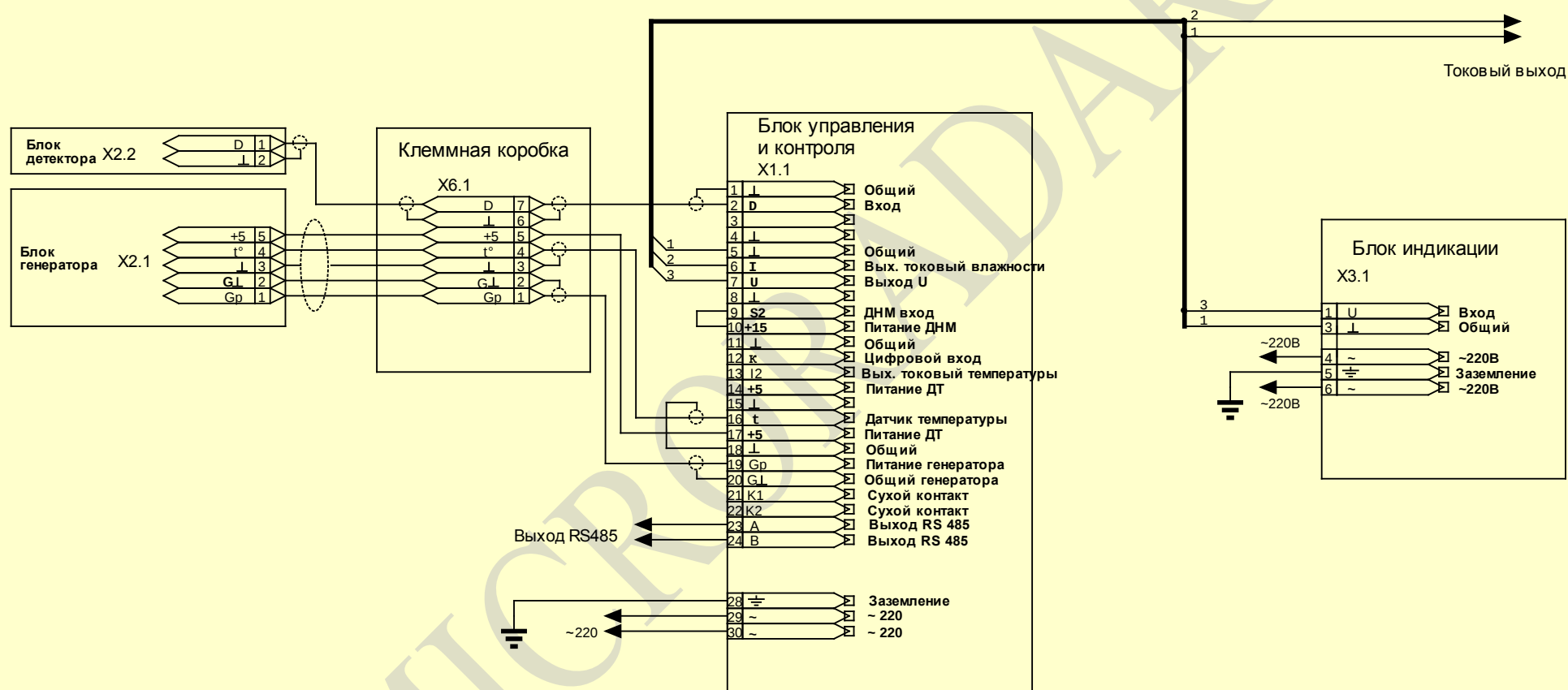
«Микрордар-113АН». Схема соединений
