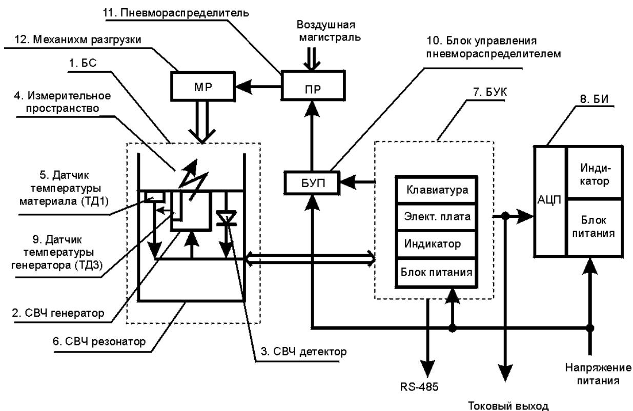
Рис. 6.3. Функциональная схема влагомера «Микрорадар-114A(D)13P»
