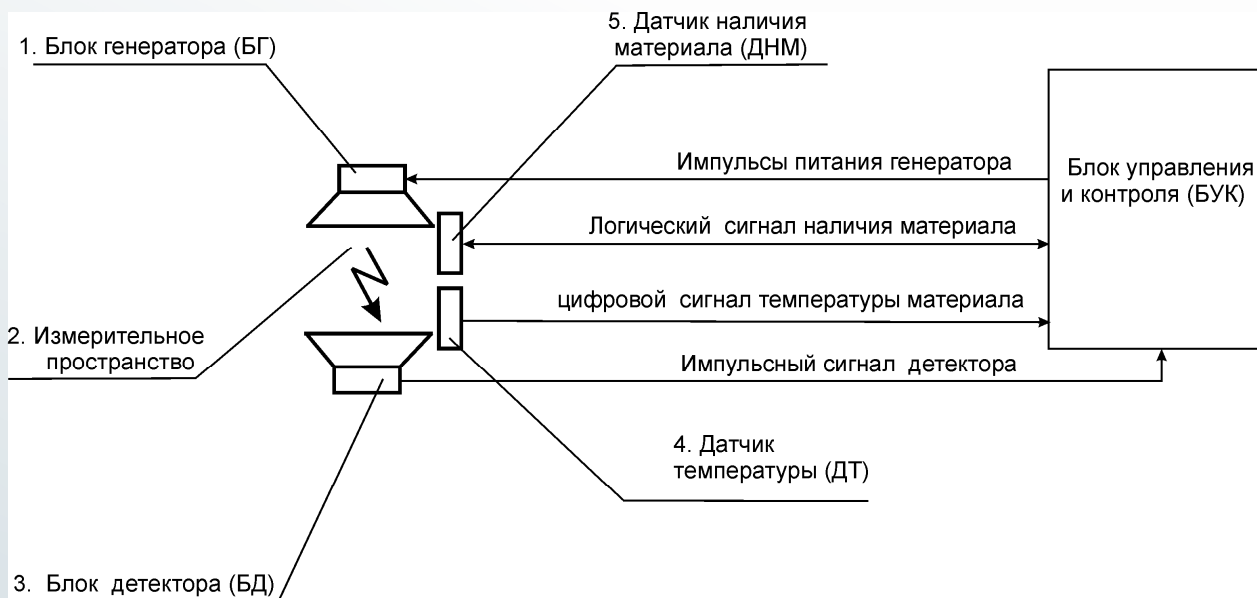
Рис. 3. Структурная схема БС и взаимодействие блоков влагомера
