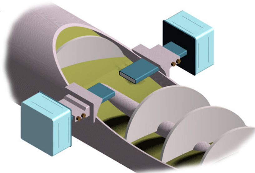
Рис. 2. Установка БС влагомера «Микрорадар-113NN» в шнековом транспортере
