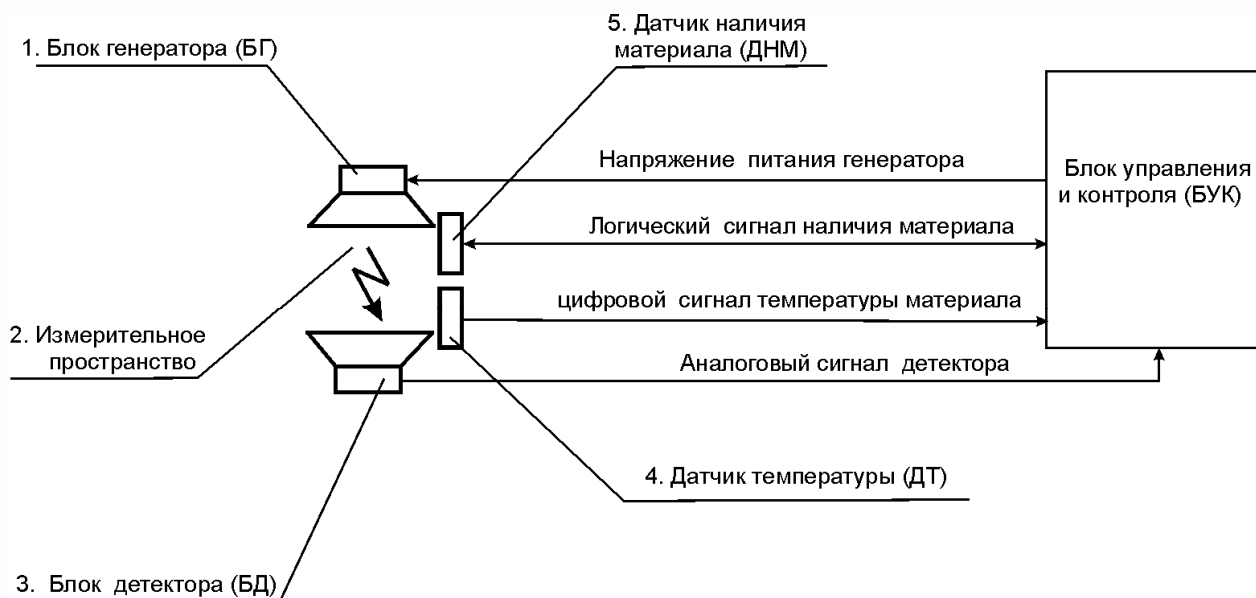
Рис. 4.2. Структурная схема БС. Взаимодействие блоков влагомера
