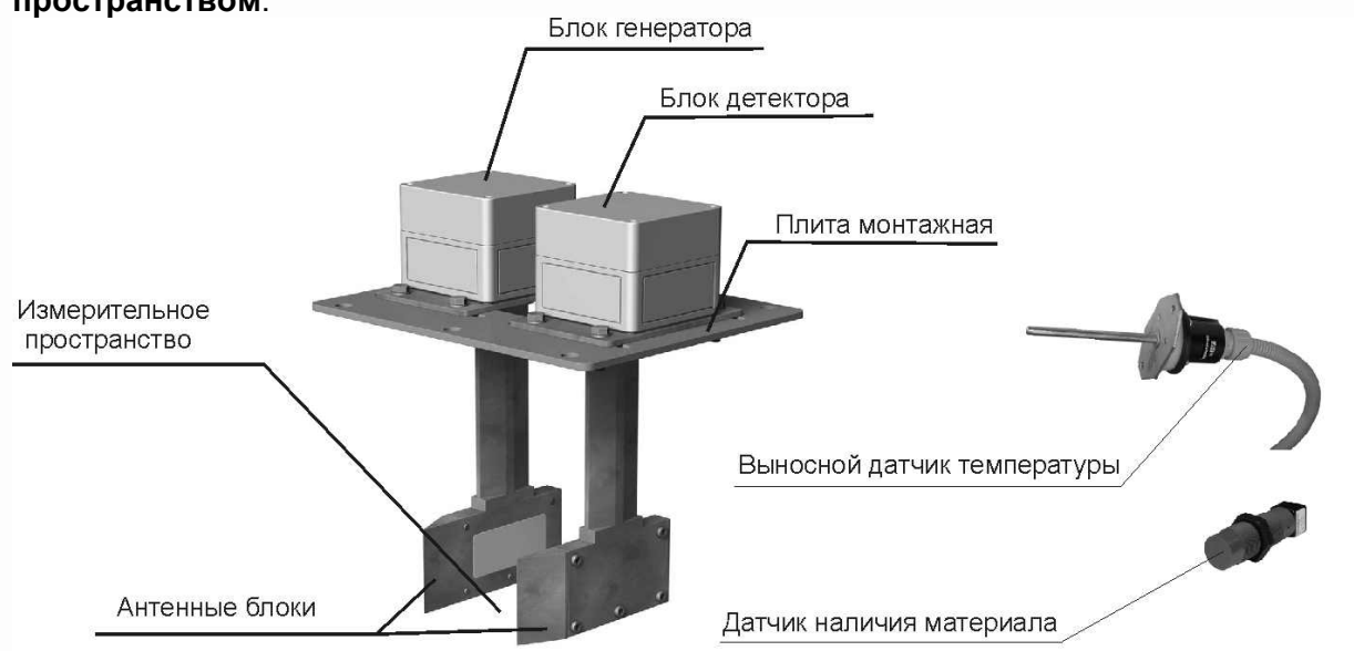
Рис. 4.1. Внешний вид блока сенсоров
